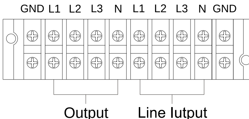
30K (L) 端子布线图
