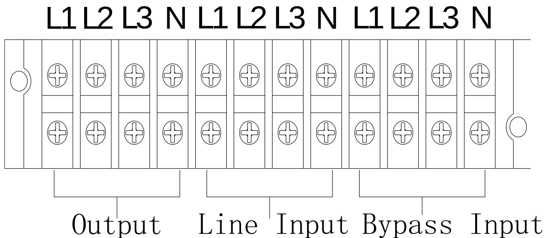
10K (L) , 20K (L) 端子布线图
