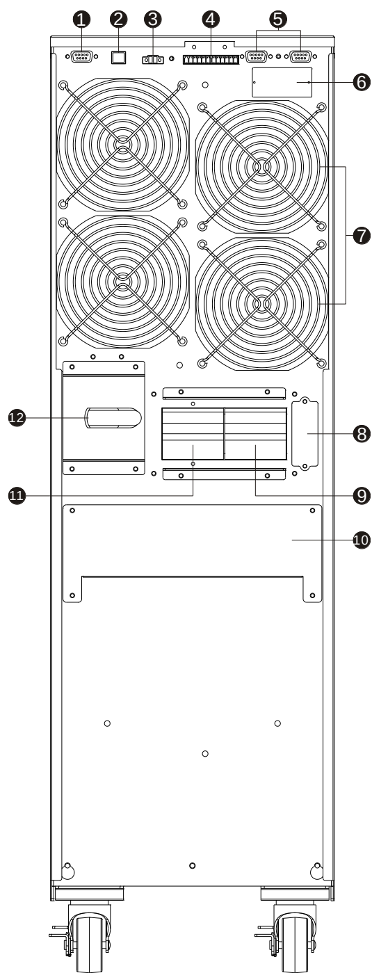
图 1: 10K(L)/15K(L)/20K(L)背板图
