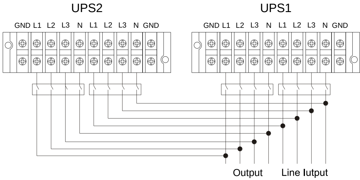
30K(L)并联系统布线图
