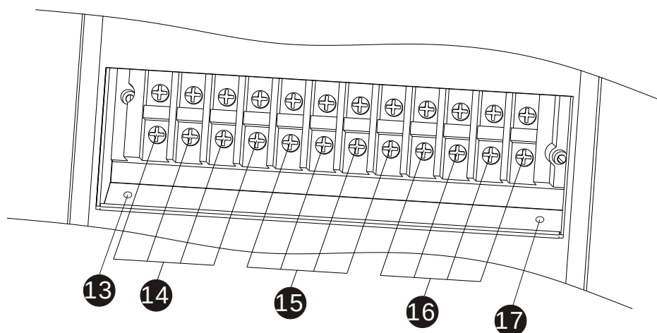
图 3: 10K(L)15K(L)/20K(L) 输入/输出端子台
