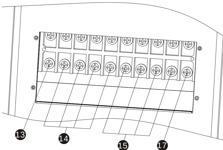
图 4: 30K(L) 输入/输出端子台
